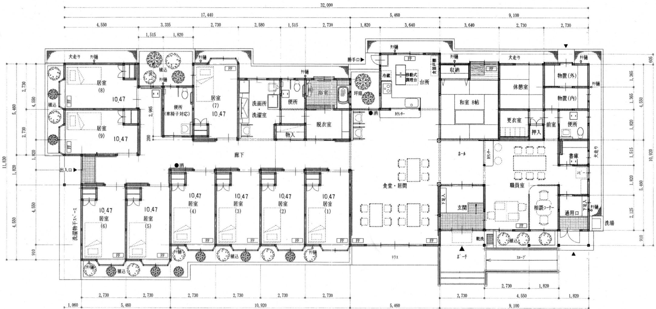
平面図 S=1/100
